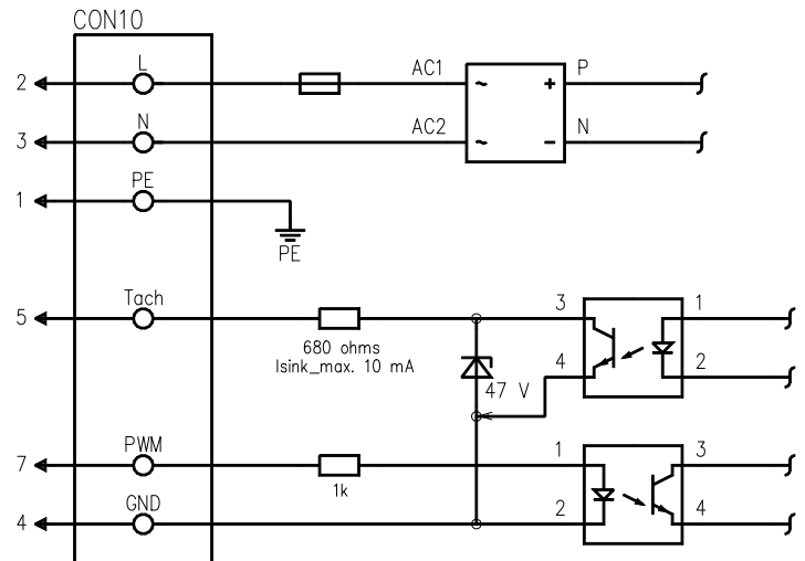
Fan/Motor
