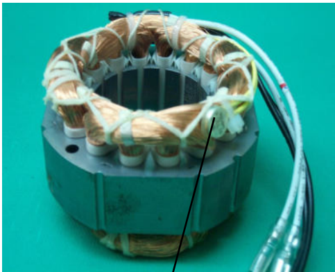
Thermal Cutout
