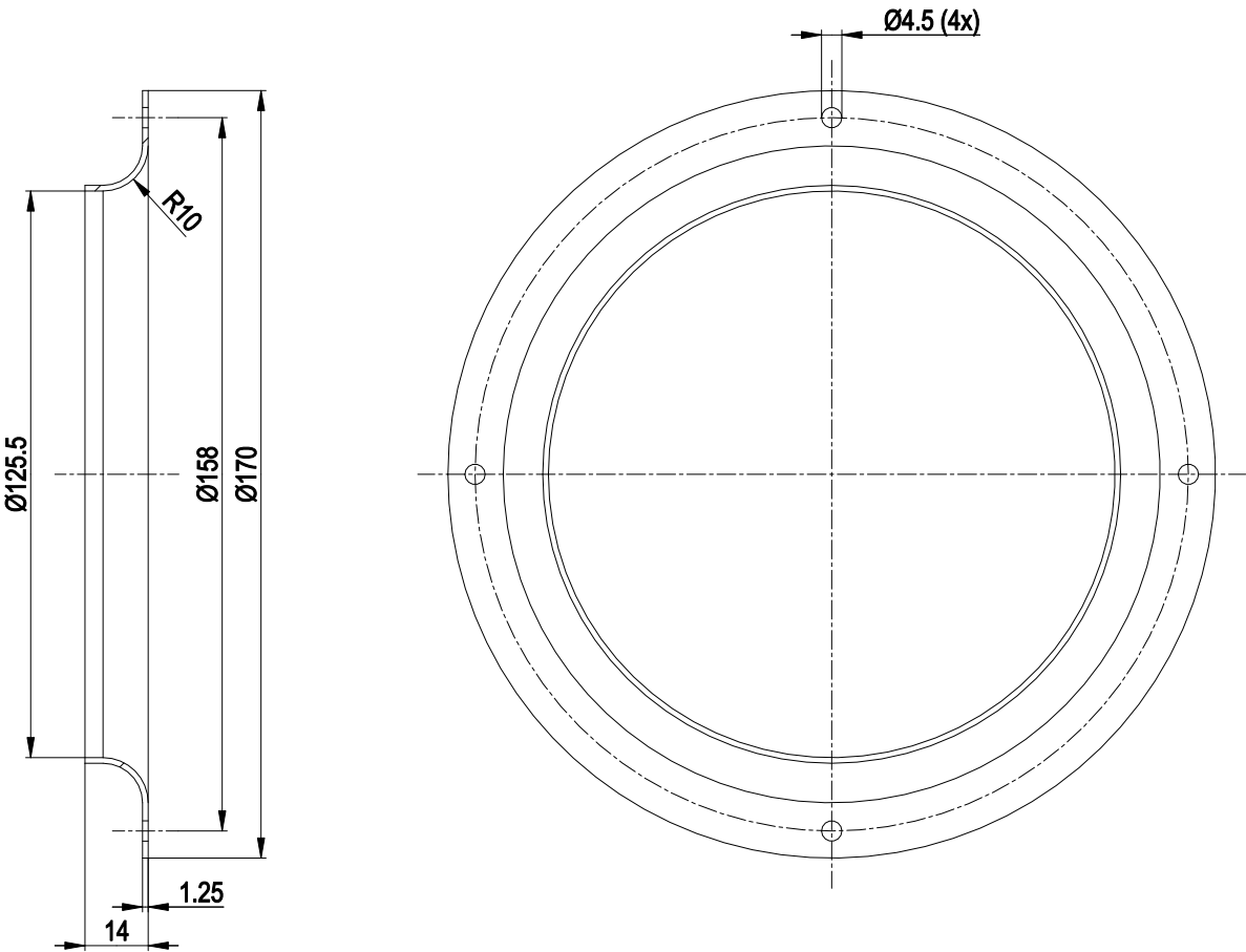
Inlet ring 09576-2-4013
